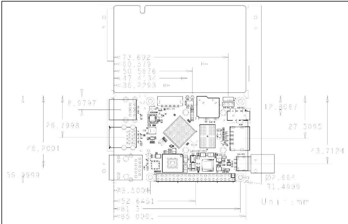
图 3.3-1 鲁班猫 1 机械尺寸图
