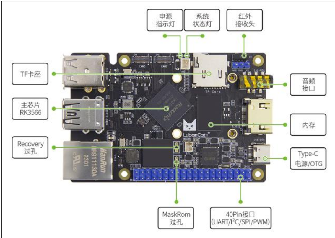
图 3.2.1-5 鲁班猫 1-V2 正面视图 2
