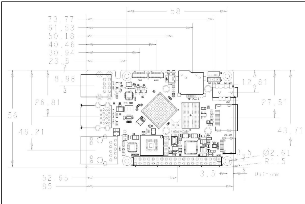
图 3.3-2 鲁班猫 1-V2 机械尺寸图
