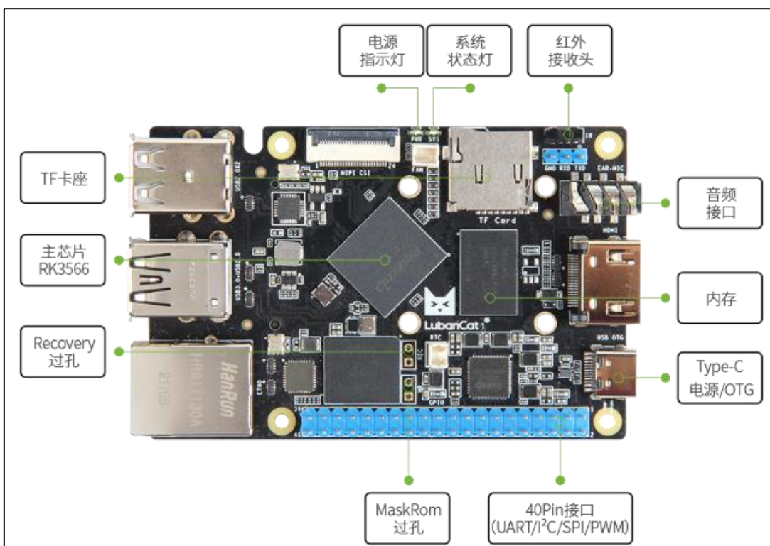
图 3.2.1-2 鲁班猫 1 正面视图 2
